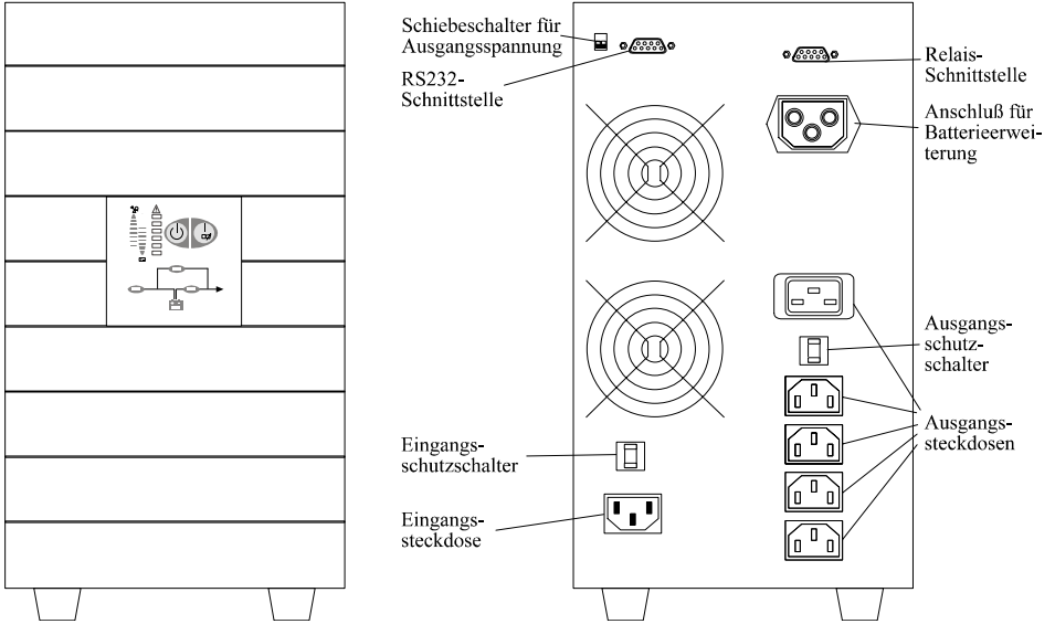
Abbildung 14: Vorder- und Rückansicht XANTO S 3000
