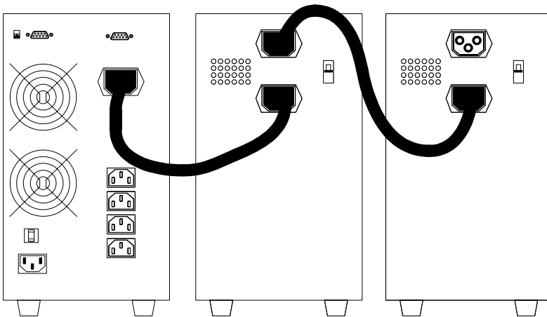
Abbildung 6: Anschluß der Batterieerweiterungen an die XANTO S 2000 und XANTO S 3000
