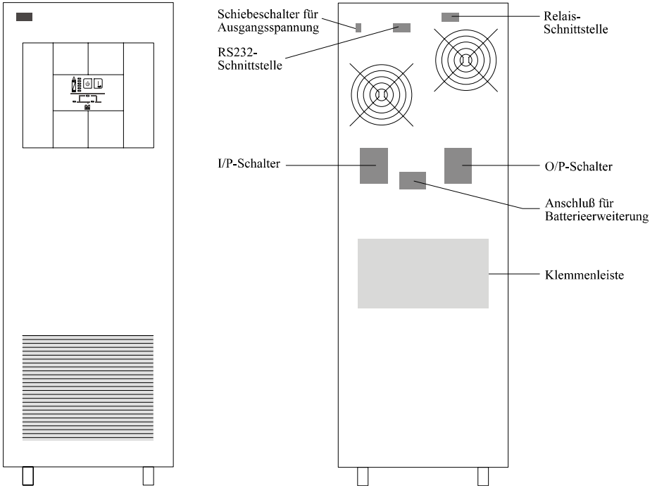
Abbildung 15: Vorderansicht und Rückansicht XANTO S 6000
