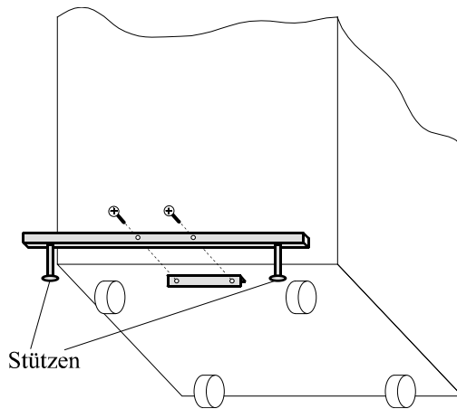
Abbildung 3: Anbringen der Standsicherung an der XANTO S 6000
