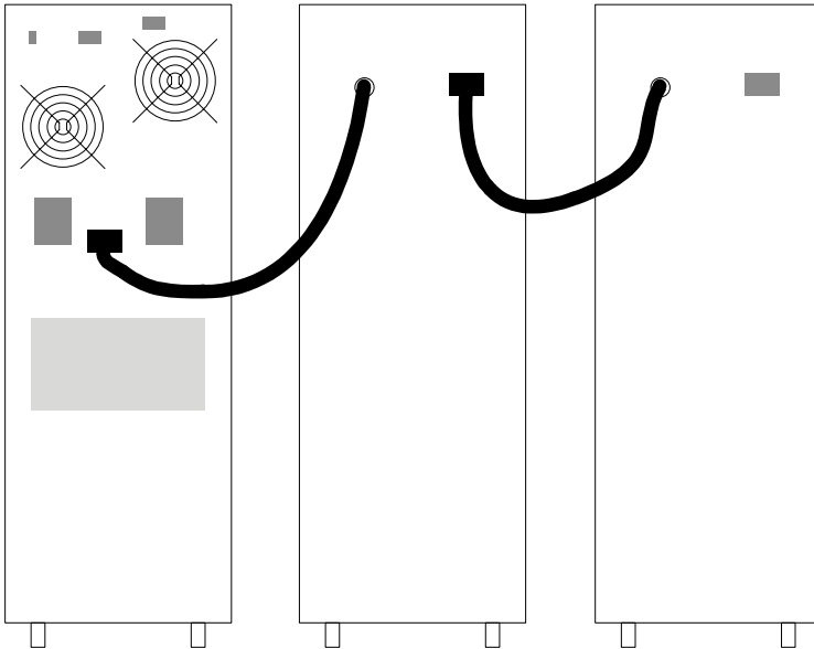
Abbildung 7: Anschluß der Batterieerweiterungen an die XANTO S 6000
