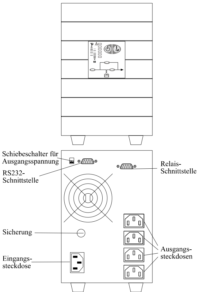
Abbildung 9: Vorder- und Rückansicht XANTO S 700
