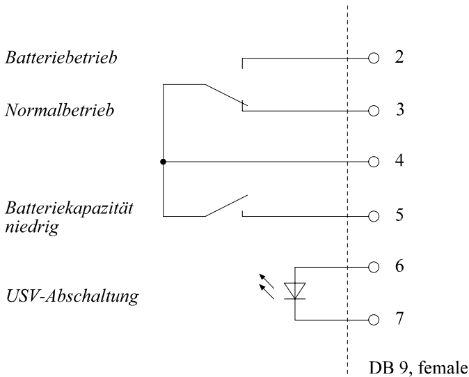
Abbildung 8: Schaltplan Relais-Schnittstelle
