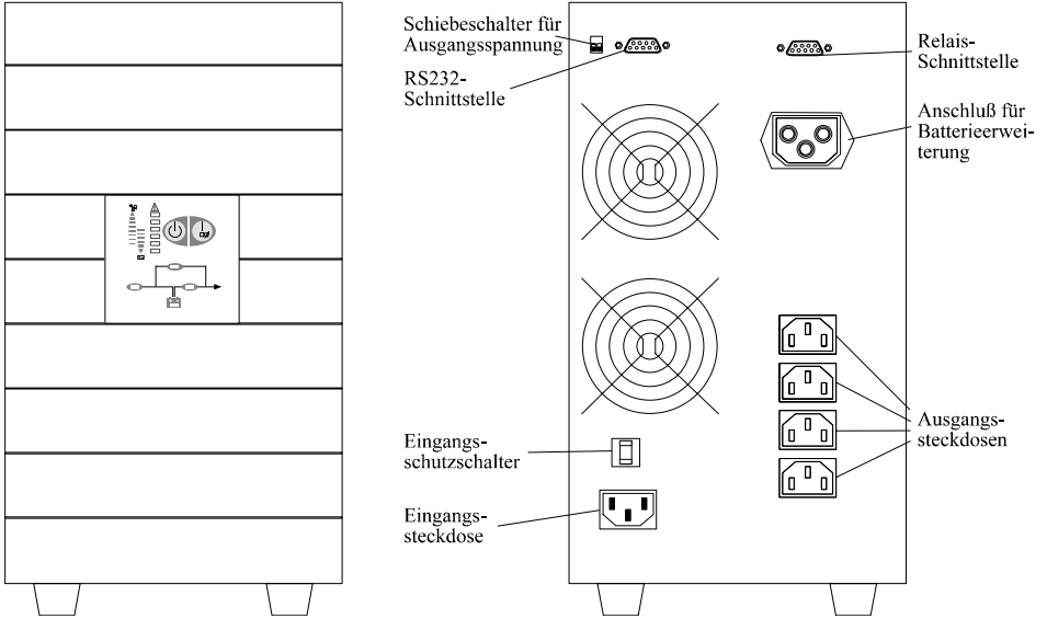
Abbildung 12: Vorder- und Rückansicht XANTO S 2000
