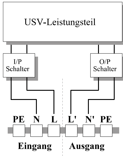
Abbildung 4: Anschlußplan XANTO S 6000.
