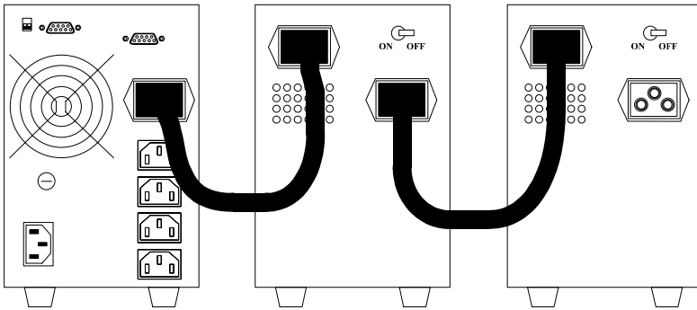
Abbildung 5: Anschluß der Batterieerweiterungen an die XANTO S 1000 und XANTO S 1500
