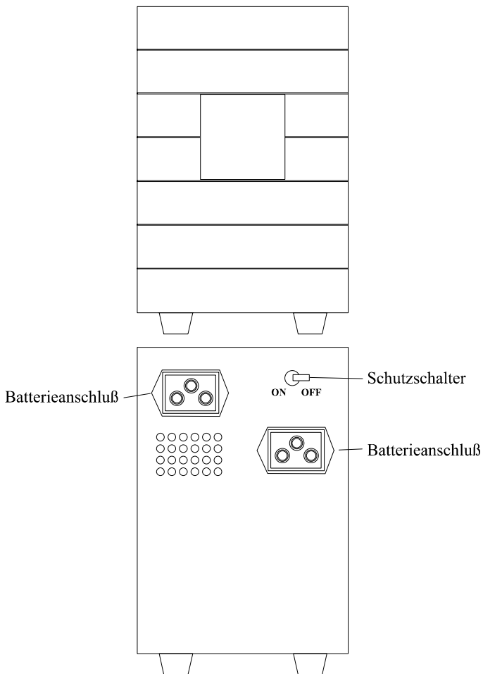
Abbildung 11: Vorder- und Rückansicht Batterieerweiterung für XANTO S 1000 und XANTO S 1500
